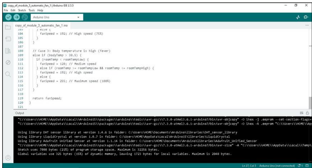
Figure 12. Arduino IDE
