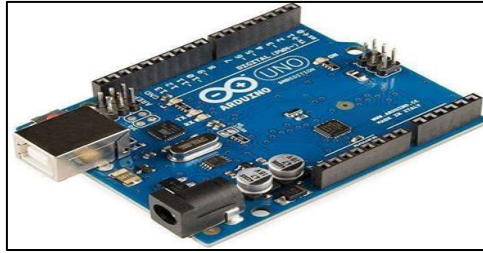
Figure 4. Arduino UNO
